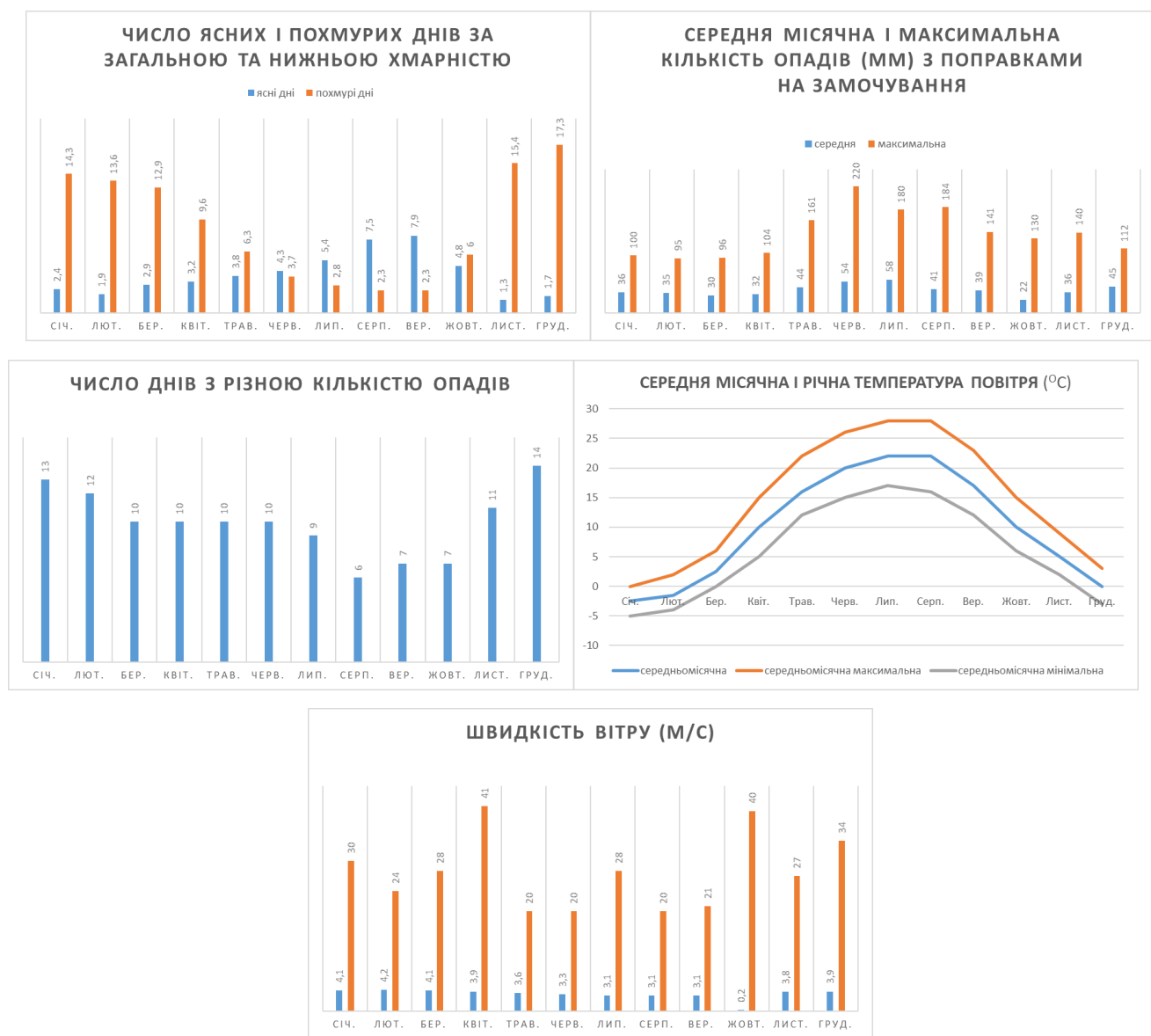
Рисунок 2.2 – Метеорологічні характеристики
